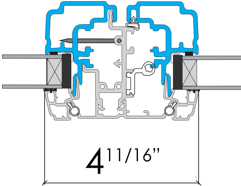
ASTRAGAL
