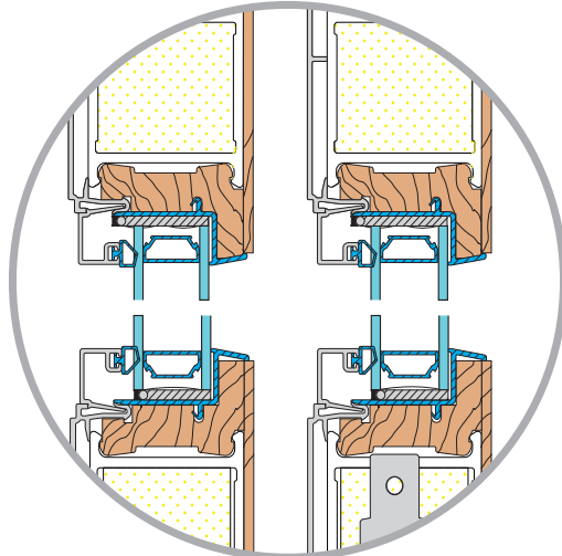
Porte levante - coulissante
